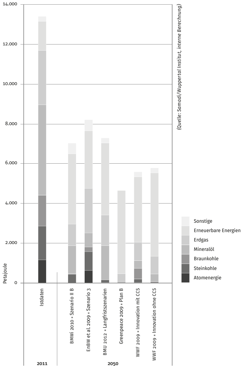
Abbildung 1: Vergleich des Primärenergieverbrauchs 2011 mit repräsentativen deutschen Szenarien für 2050 nach Energieträger (in Petajoule pro Jahr).
