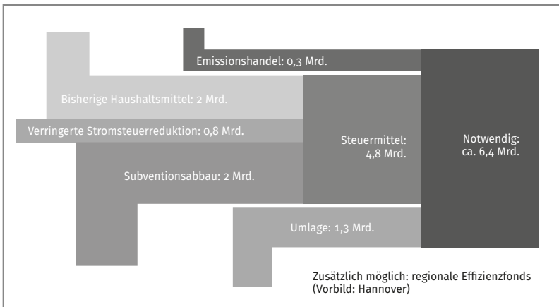
Abbildung 9: Vorgeschlagenes Finanzierungskonzept für das Erreichen der Einsparziele.
